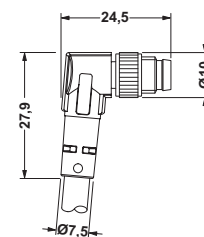
Hane M 8 x 1, vinklat utförande
