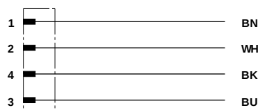
Anslutna M 8-kontakter
